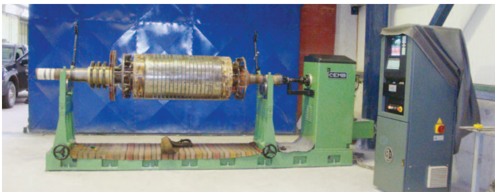
ΖΥΓΟΣΤΑΘΜΙΣΗ ΔΡΟΜΕΑΣ -ΗΛΕΚΤΡΟΚΙΝΗΤΗΡΑ
